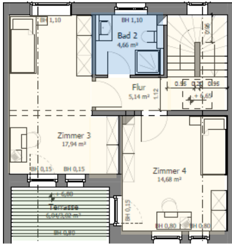
2. OG
